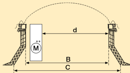
SIMPLE MOTEUR
